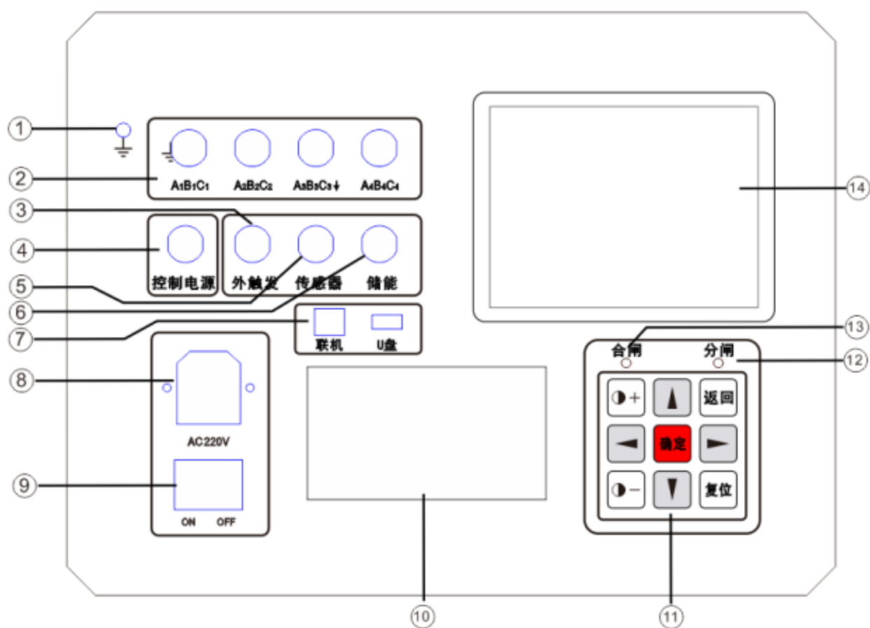
图1 面板布局图
