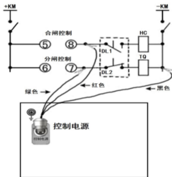
图 12 分合闸控制线接线图
