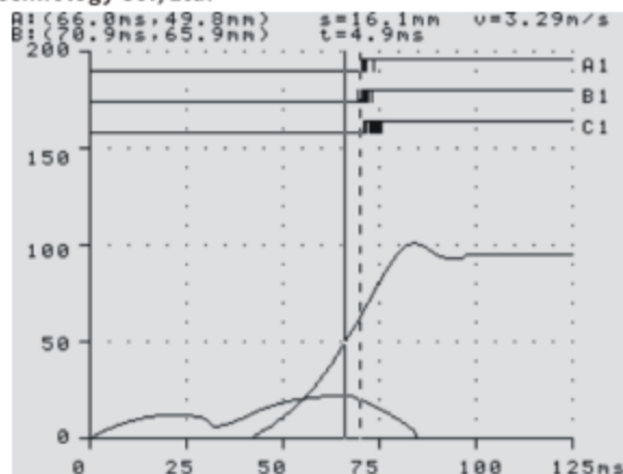
图6 时间-行程数据曲线图
