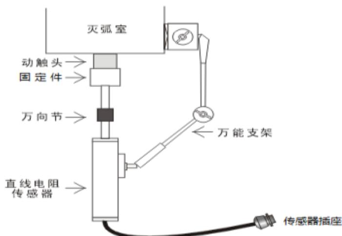
图 14 行程传感器安装示意图
