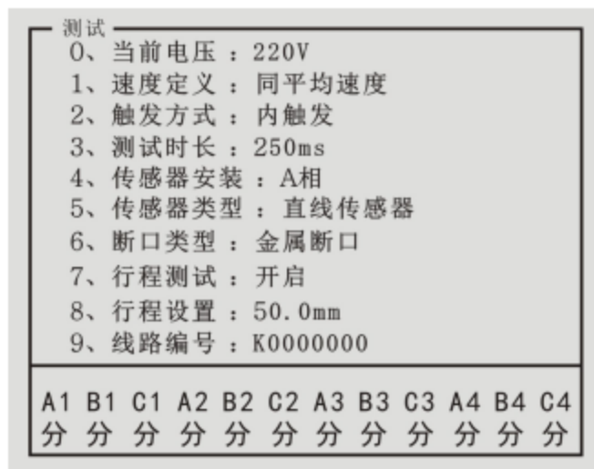
图 15 断口状态示意图
