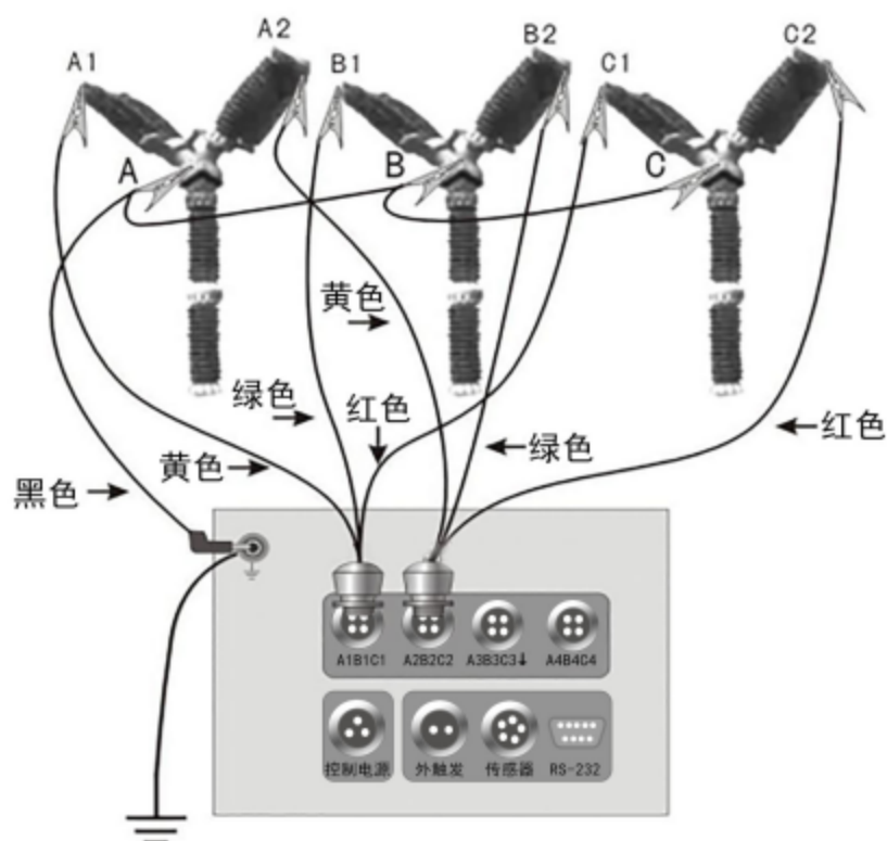
图 10 六断口接线
